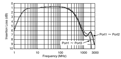
2) #458PT-1586 (Impedance Ratio=50Ω:200Ω)
