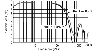
4) #458PT-1565 (Impedance Ratio=50Ω:200Ω)
