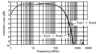
3) #458PT-1587 (Impedance Ratio=50Ω:200Ω)
