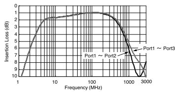
1) #458PT-1619 (Impedance Ratio=50Ω:200Ω)
