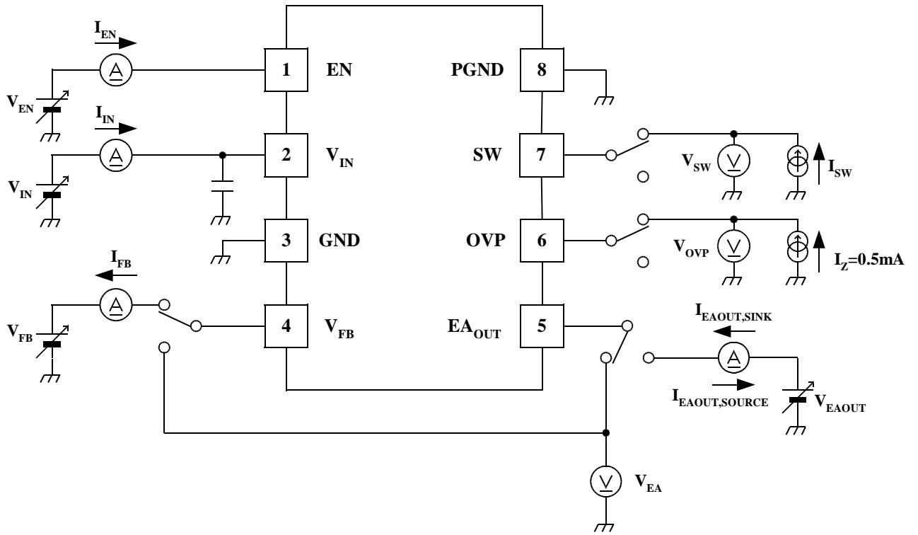
測定回路図
